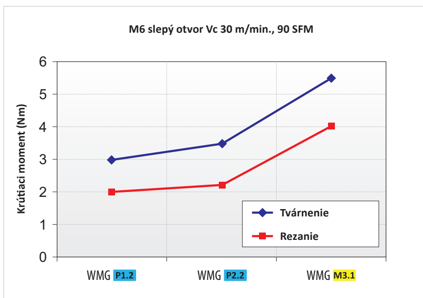
Porovnanie krútiaceho momentu medzi tvárniacimi a rezačmi závitníkmi v rôznych skupinách materiálov.
